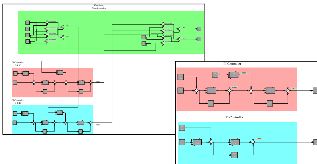
Rotor y controladores de red PWM
